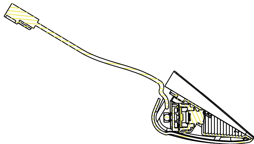
リアカメラ車内設置ブラケット
